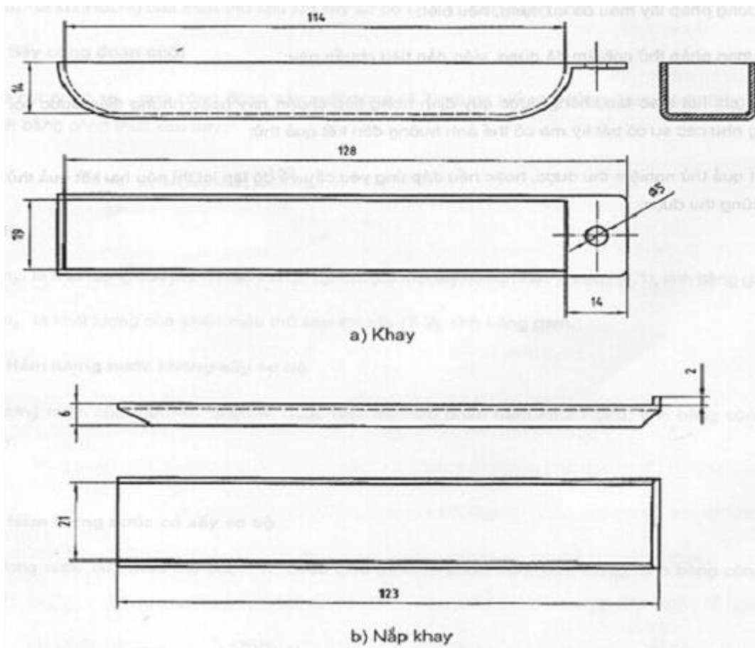
Hình A.1 - Hình vẽ của khay kim loại và nắp thích hợp (chỉ để tham khảo)
